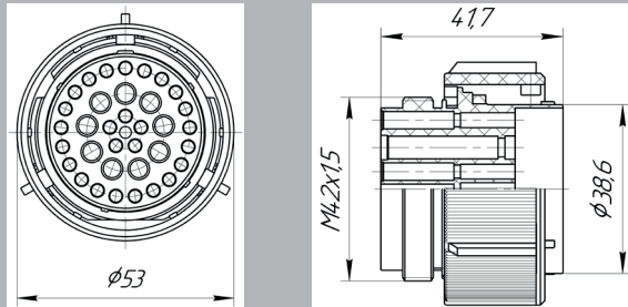
Вилка СЦБ-35В
