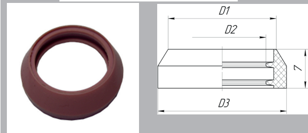
Втулка
