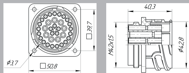
Розетка СЦБ-35Р.01
